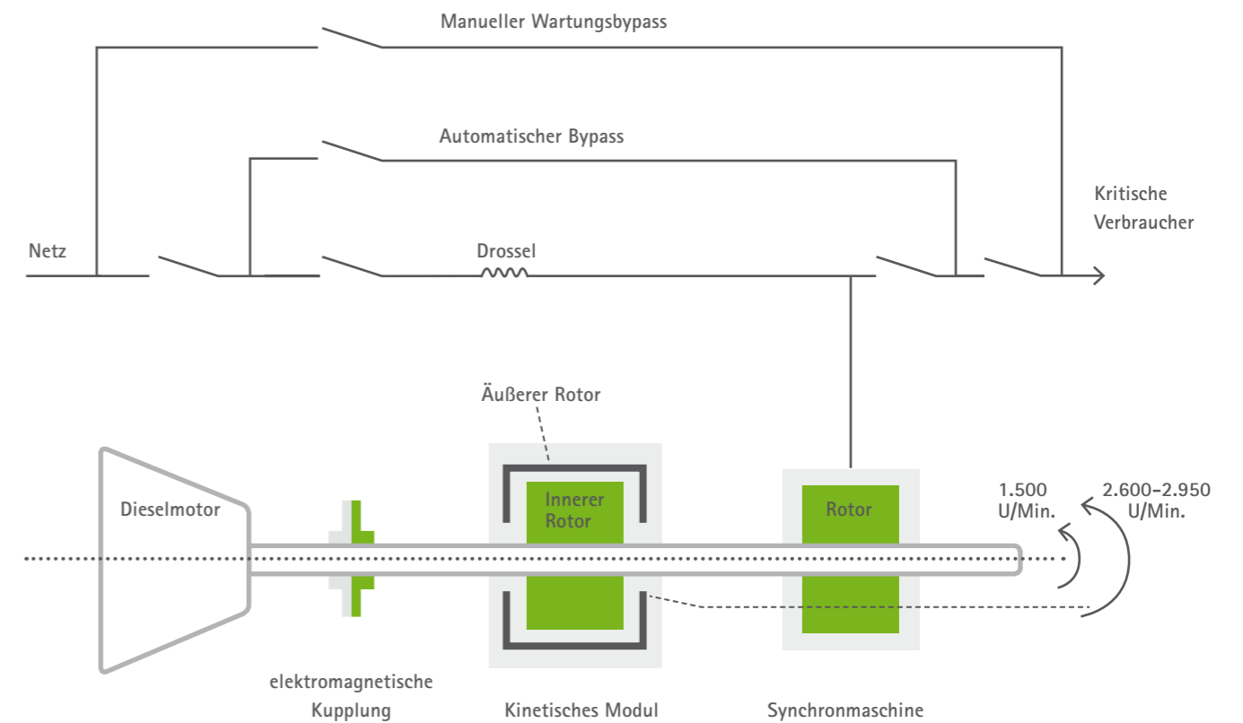
Abb. 5.5: Prinzipielle Darstellung eines dieseldynamischen USV-Systems
